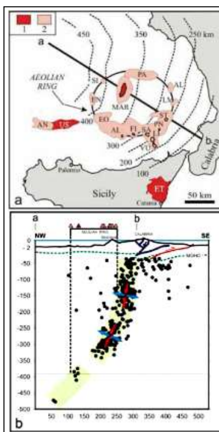
Fig. 5: Geometria del Piano di Benjoff nel Tirreno Meridionale. (da Bell K. et al. (2005). Reasoning and beliefs about Italian geodynamics. Boll. Soc. Geol. It. , 5, 119-127). Legenda: PA) Palinuro; AL) Alcione; LM) Lametini; ST) Stromboli; PN) Panarea; SA) Salina; LI) Lipari; VU) Vulcano; FI) Filicudi; AL) Alicudi; EO) Eolo; EN) Enarete; SI) Sisifo; MAR) Marsili; AN) Anchise; US) Ustica; ET) Etna
