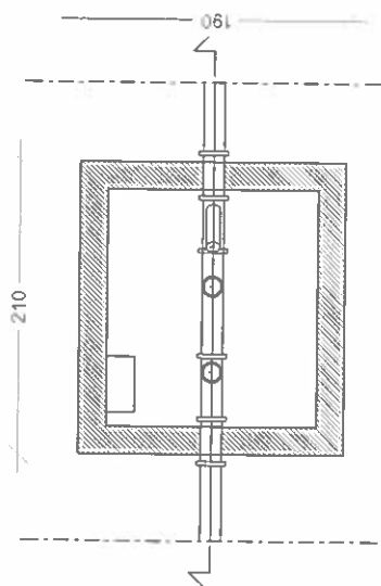
particolare pozzetto per le ispezioni
