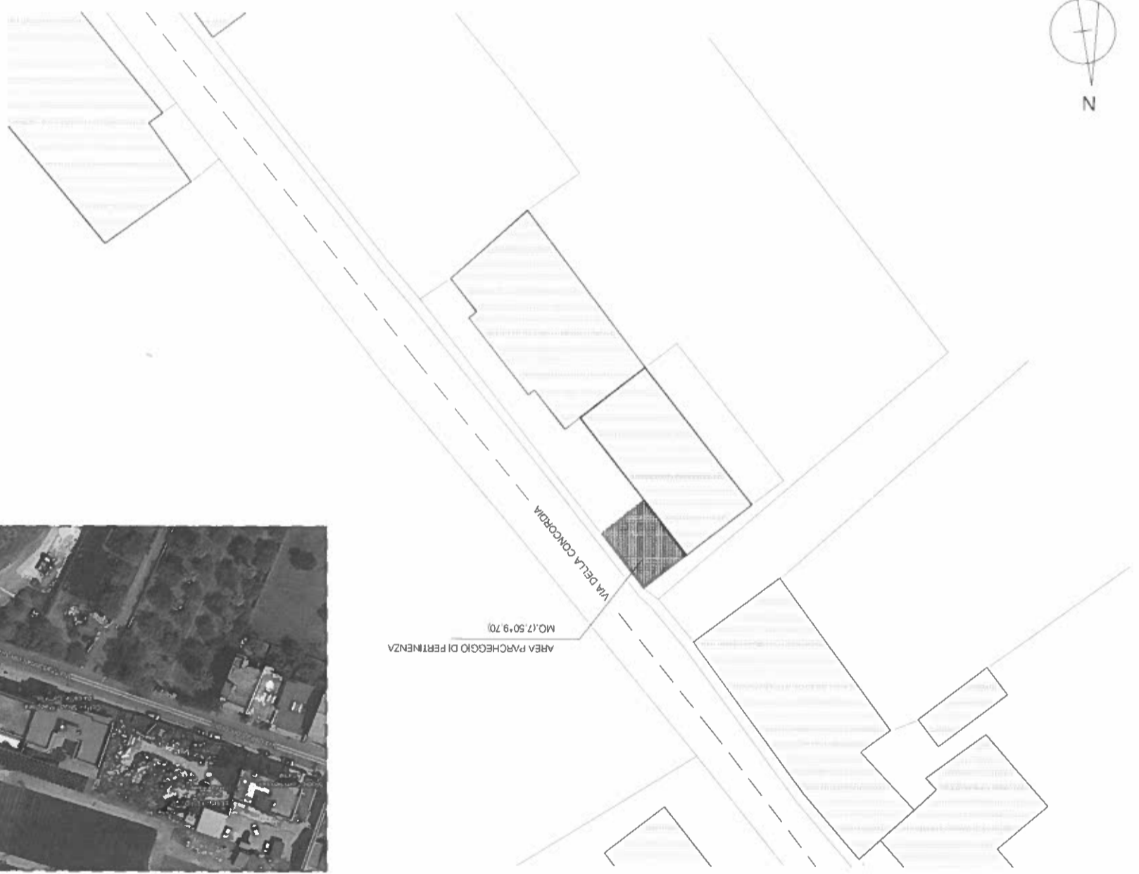
PLANIMETRIA GENERALE Rappr. 1:500
