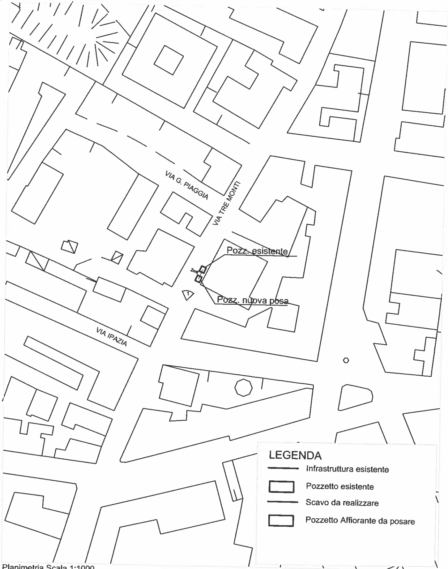
Planimetria Scala 1:1000
